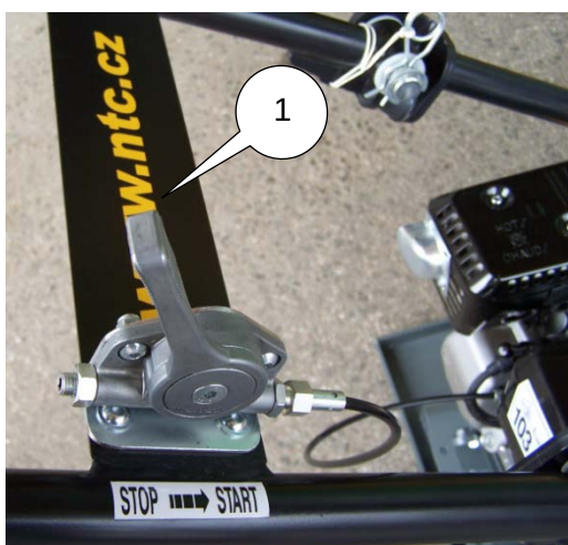
Obr. Páka plynu v poloze „volnoběh“
